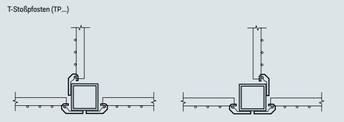
T-Stoß-Anbindung links oder rechts - beide Anbindungen vorhanden.
